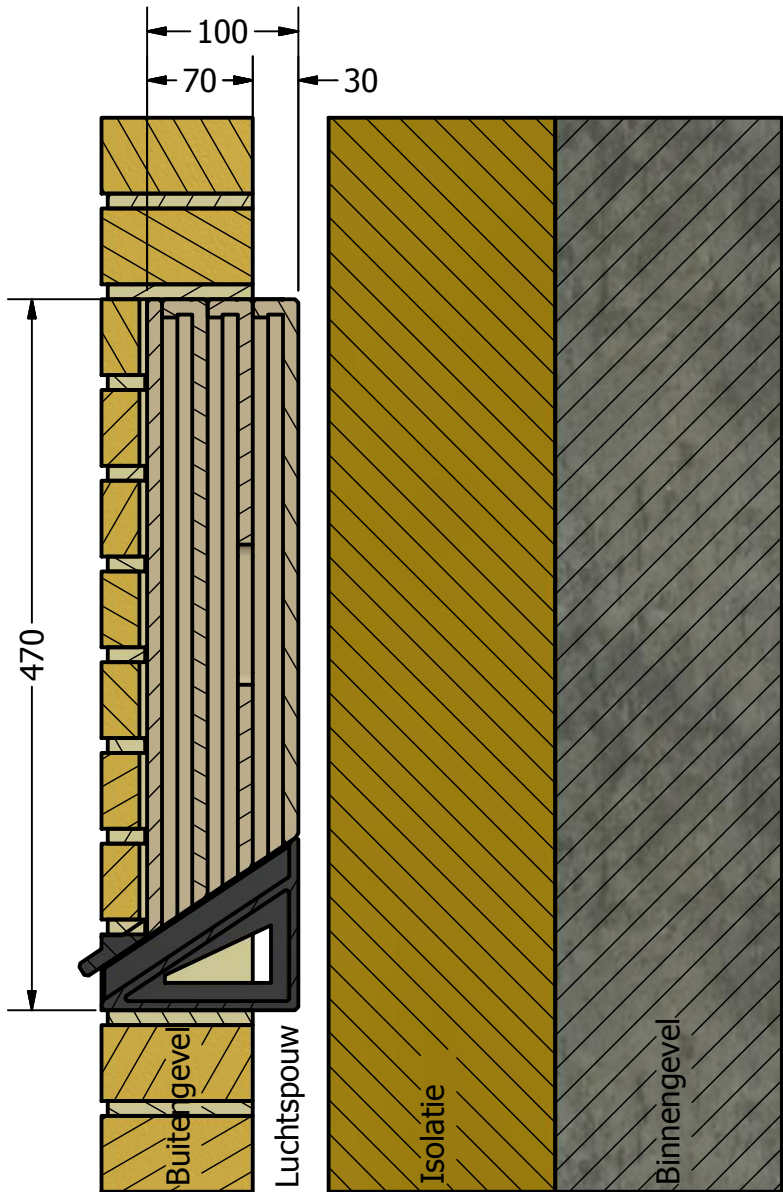
Principe dwarsdoorsnede spouwmuur
