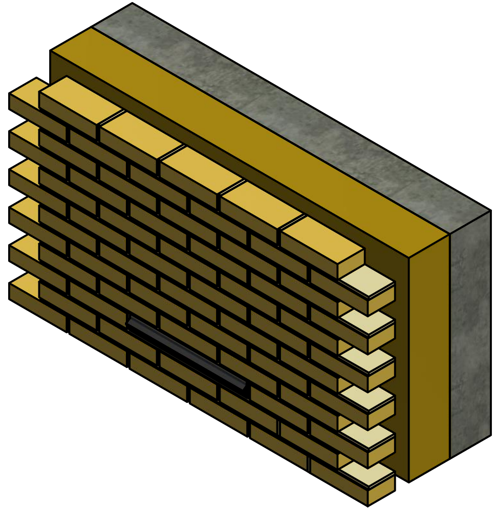
Principe spouwmuur impressie
